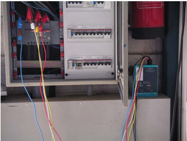
Fig. 2.- Memobox 300 smart installation
