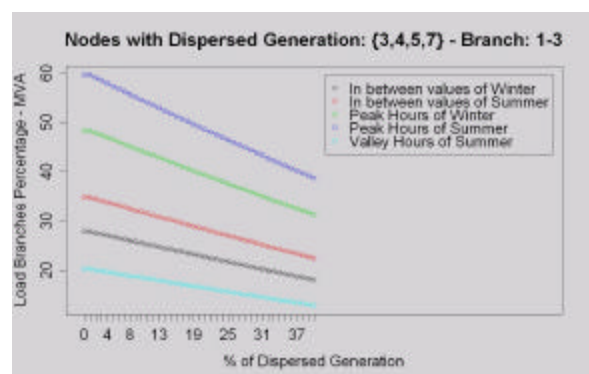
Fig. 21. HV Network – Load Branches
